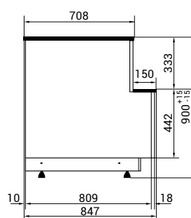
▼ neutrální pult
