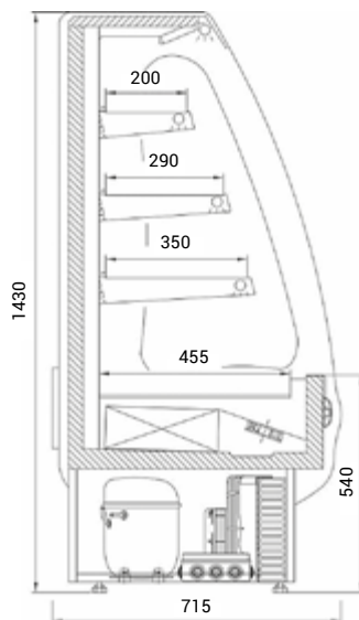
bokorys Piccoli
