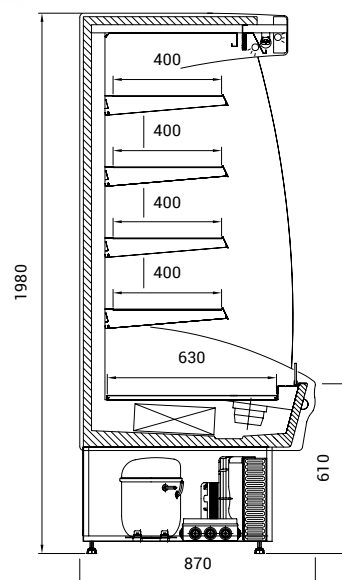
bokorys Martini 90
