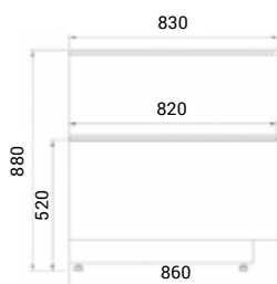
neutrální pult
