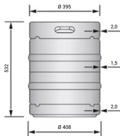
bokorys sud KEG 50 l
