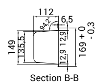
► IC 400 SCE
