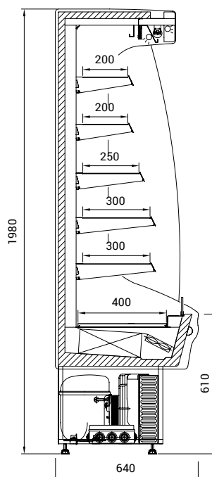
bokorys Mini Martini 65
