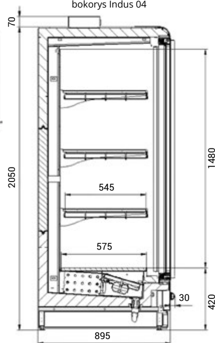
bokorys Indus 04
