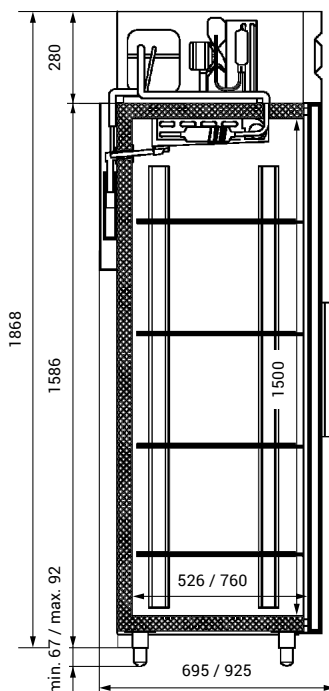
▼ CM 114 – skříň s neodděleným vnitřním prostorem
