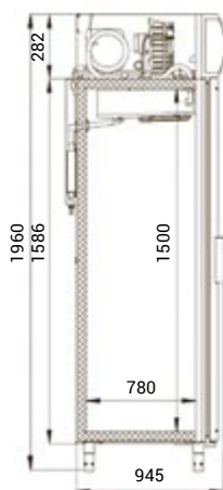
bokorys DM 107
