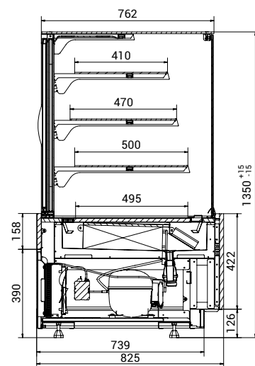
▼ Juka Lumina
