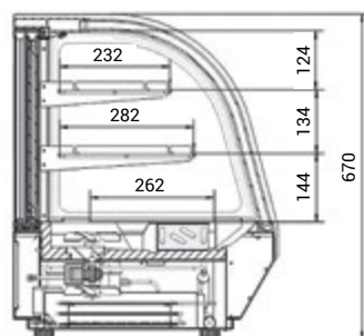
▲ boční pohled
