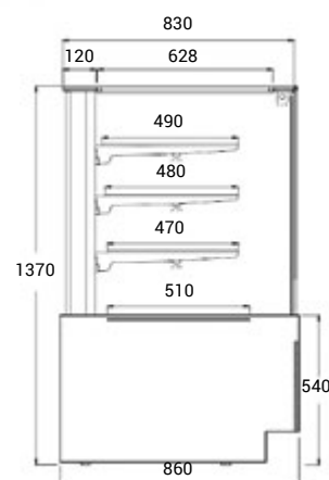
bokorys Rafaello
