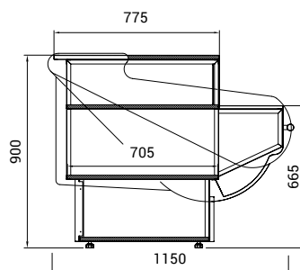
▼ neutrální pult
