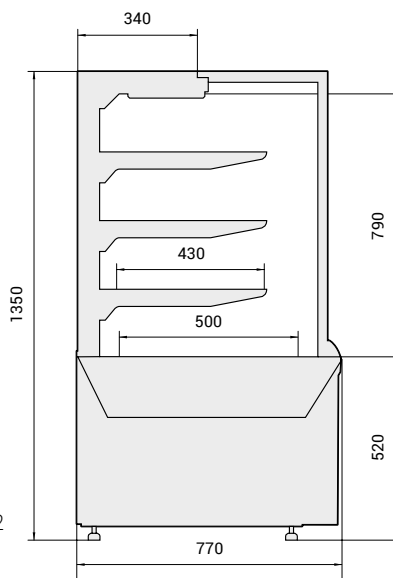
Carina 06 bokorys
